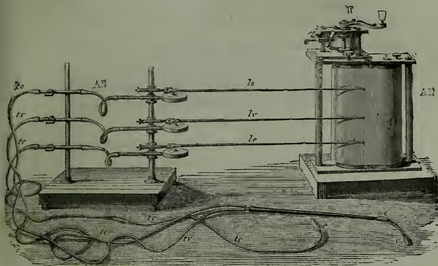
FIG. 67. — Appareil enregistreur.
